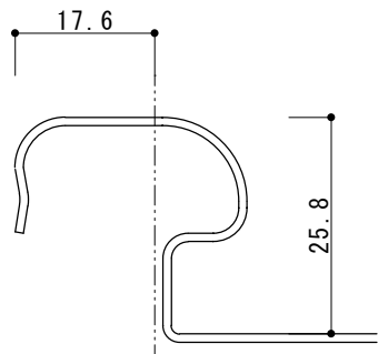
A部詳細
