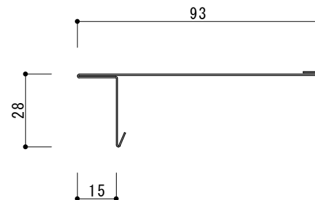
唐草93幅 断面形状 S=1/2
