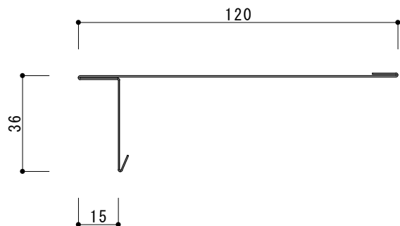
唐草120幅（広幅）断面形状 S=1/2
